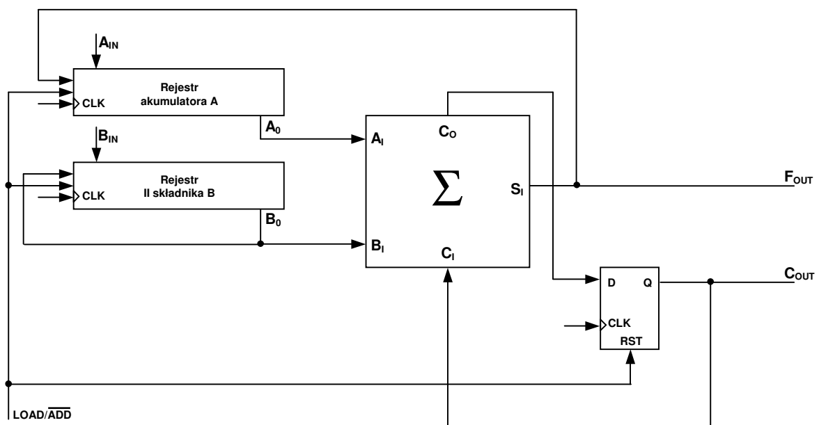
Schemat sumatora akumulującego
